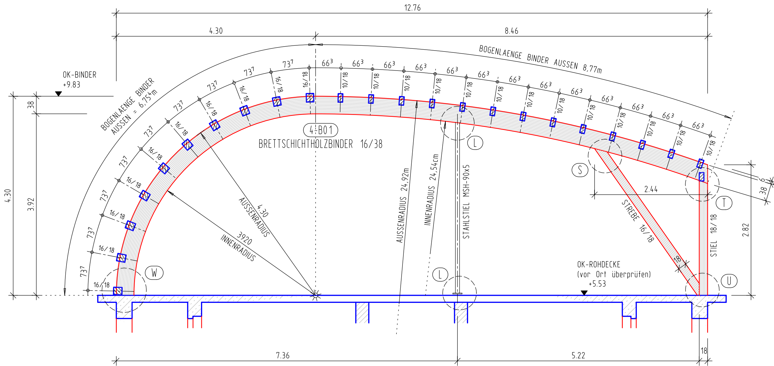
SCHNITT 4-B M1:50
